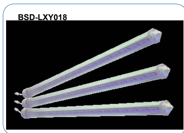
外形尺寸图 Dimension Diagram
